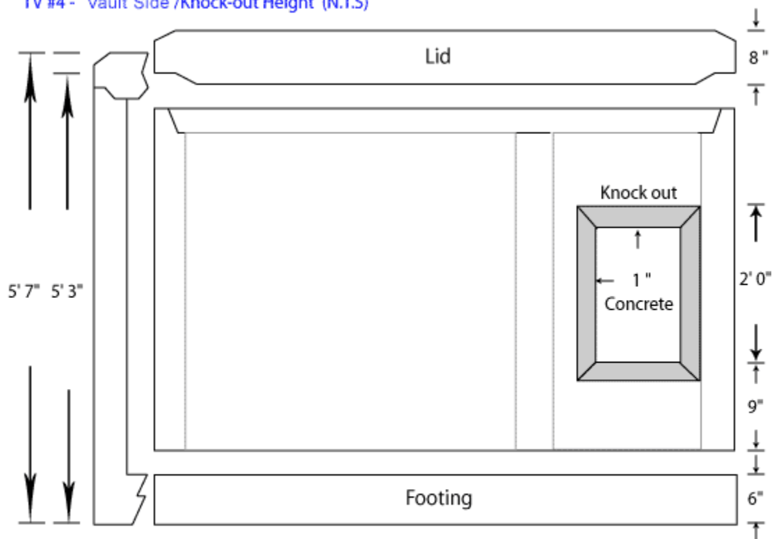
TV #4 - Vault Side / Knock-out Height (N.T.S)
